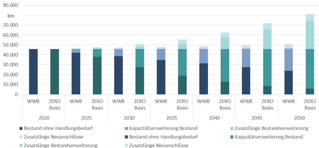
Bild A.2 Vergleich der Entwicklung der Leitungslängen der NE 5 der Szenarien WWB und ZERO Basis im zeitlichen Verlauf von 2020 bis 2050
