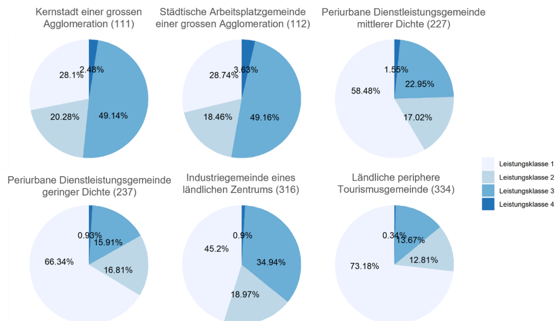
Bild 3.16 Anteil der Leistungsklassen an installierter Leistung im Jahr 2050 im Szenario ZERO Basis für die ausgewählte Gemeindetypen (Leistungsklasse 1: \leq 30 kWp; Leistungsklasse 2: 30-100 kWp; Leistungsklasse 3: 100-1000 kWp; Leistungsklasse 4: > 1000 kWp).
