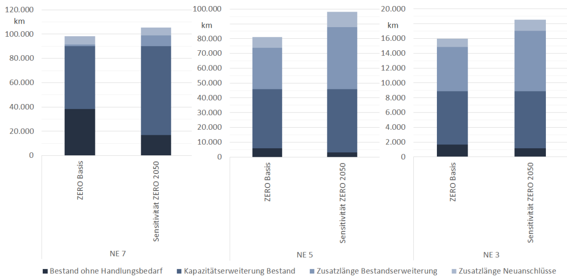
Bild 3.24 Ergebnisse der Sensitivität ZERO 2050 für das Jahr 2050 im Vergleich zum Szenario ZERO Basis (Leitungsebenen NE 7, NE 5 und NE 3)
